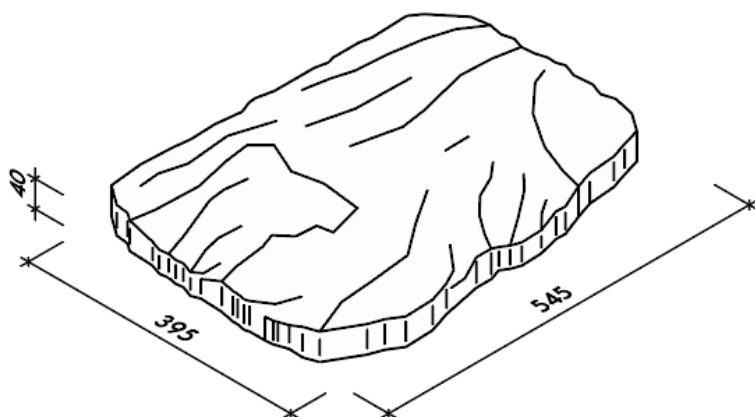
Obr. č. 10 Nášlap Břidlice V. rozměry
