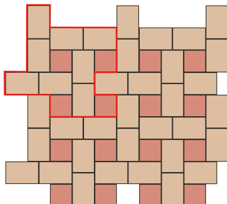
Skladba Plošná dlažba vymývaná 11
