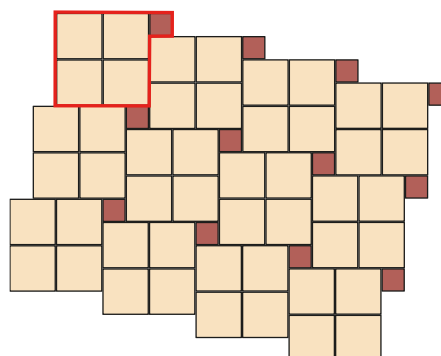
Skladba Plošná dlažba vymývaná 22
