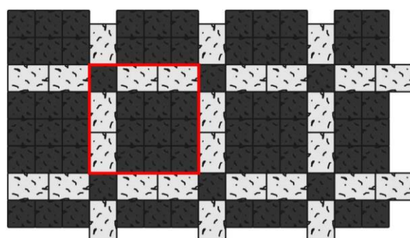
Obr. č.14 – Návrh pokládky z prvků Čtverec 12 / 12 / 4 a Obdélník 18 / 12 / 4
