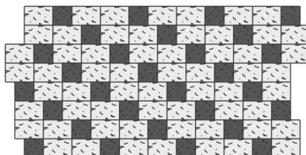
Obr. č.12 – Návrh pokládky z prvků Čtverec 12 / 12 / 4 a Obdélník 18 / 12 / 4
