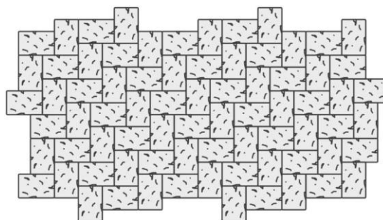
Obr. č.8 – Návrh pokládky z prvků Obdélník 18 / 12 / 4
