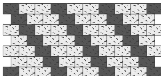
Obr. č.6 – Návrh pokládky z prvků Obdélník 18 / 12 / 4
