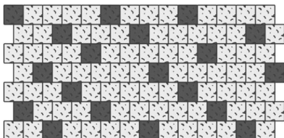
Obr. č.5 – Návrh pokládky z prvků Čtverec 12 / 12 / 4
