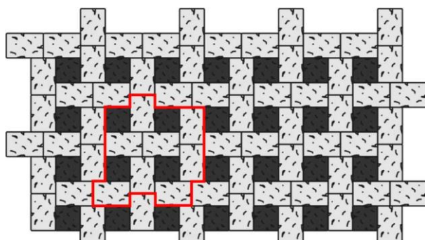
Obr. č.13 – Návrh pokládky z prvků Čtverec 12 / 12 / 4 a Obdélník 18 / 12 / 4
