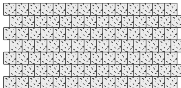
Obr. č.2 – Návrh pokládky z prvků Čtverec 12 / 12 / 4
