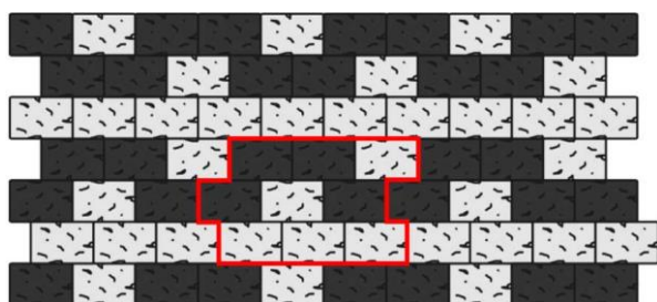
Obr. č.7 – Návrh pokládky z prvků Obdélník 18 / 12 / 4
